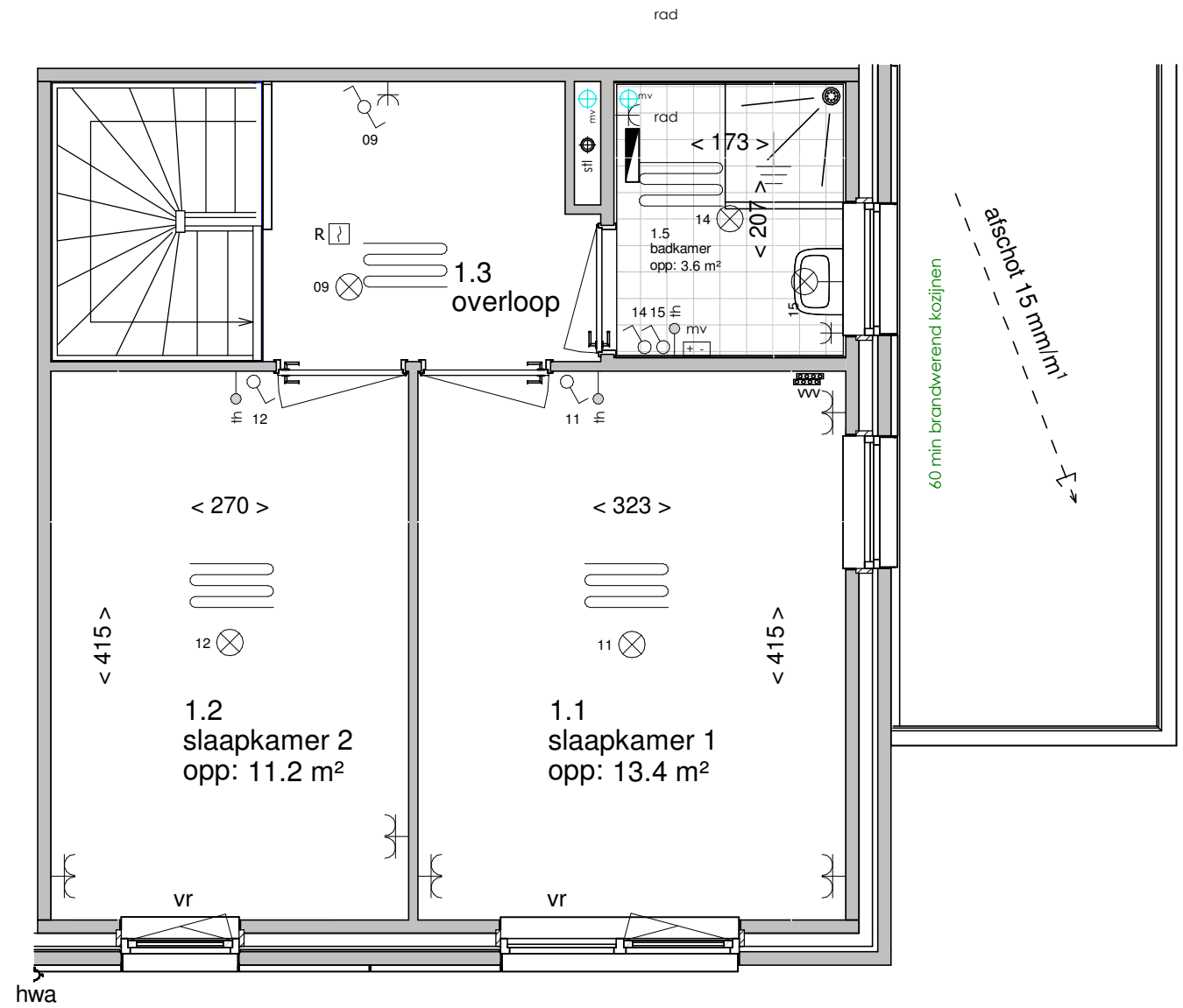
Eerste verdieping
